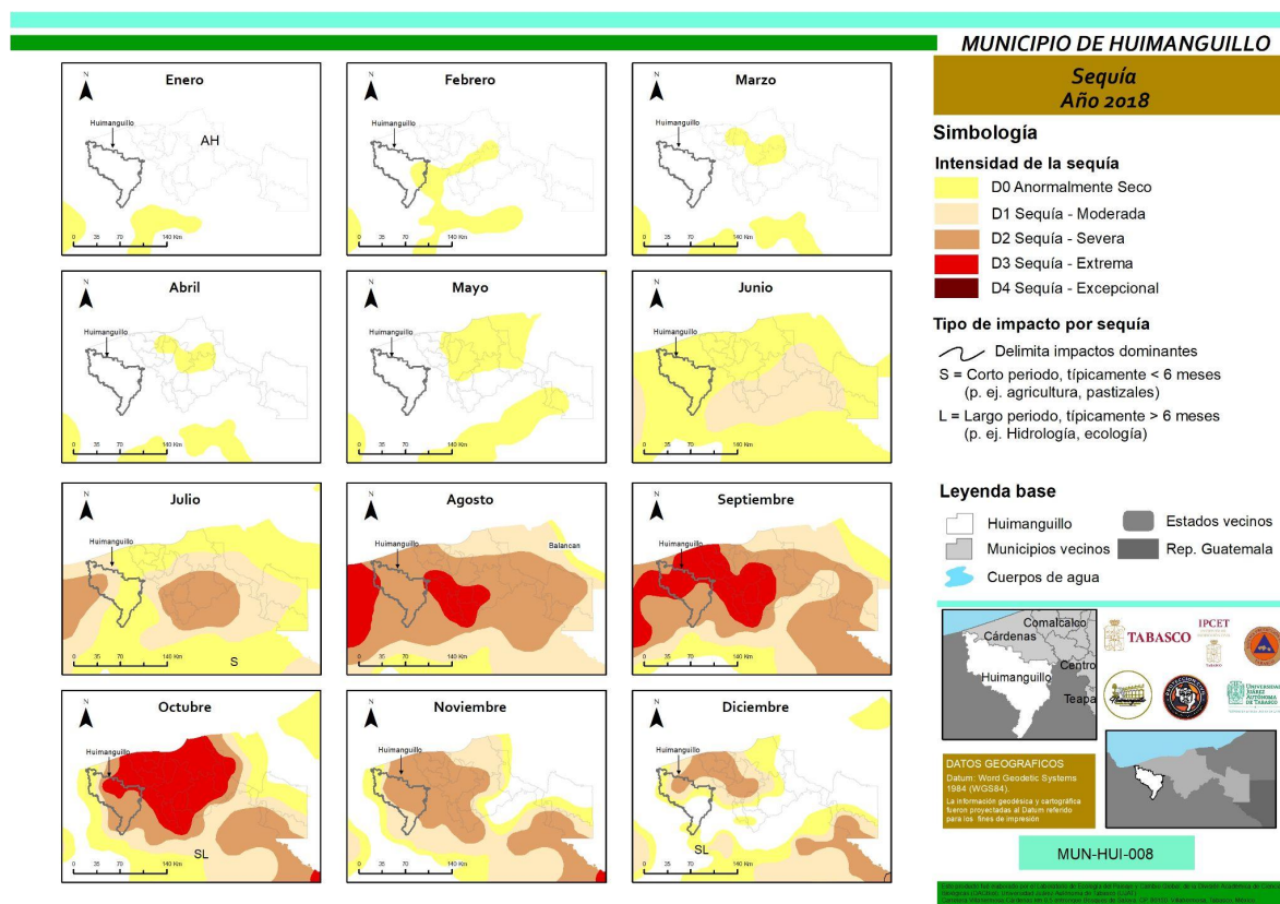
Figura 40. Categorías de sequía en el municipio de Huimanguillo durante los meses del año 2018.
