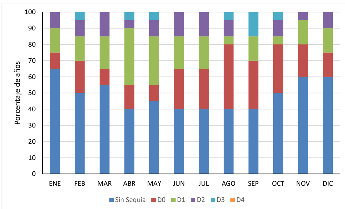
Figura 37. Ocurrancia estacional (mensual) de las condiciones de sequía en el periodo de 2003-2022. Municipio de Huimanguillo, Tabasco.
