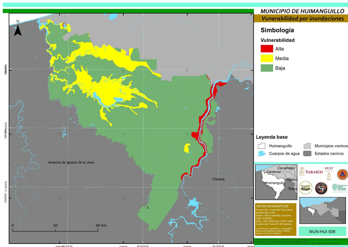
Figura 31. Zonificación del grado de vulnerabilidad a inundaciones en el municipio de Huimanguillo.
