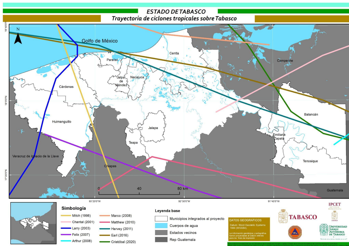
Figura 41. Trayectoria de ciclones tropicales sobre el estado de Tabasco (periodo 1980-2021).
