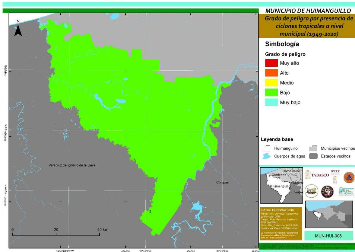
Figura 43. Grado de peligro por presencia de ciclones para el municipio de Huimanguillo.
