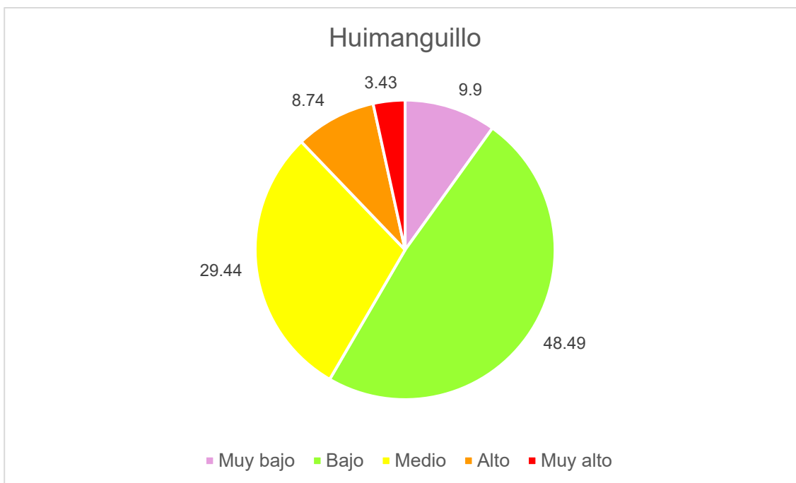
Figura 29. Proporción de la superficie municipal de Huimanguillo expuesta al peligro de inundación.
