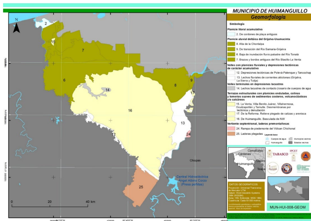
Figura 3. Mapa de Geomorfología del Municipio de Huimanguillo.
