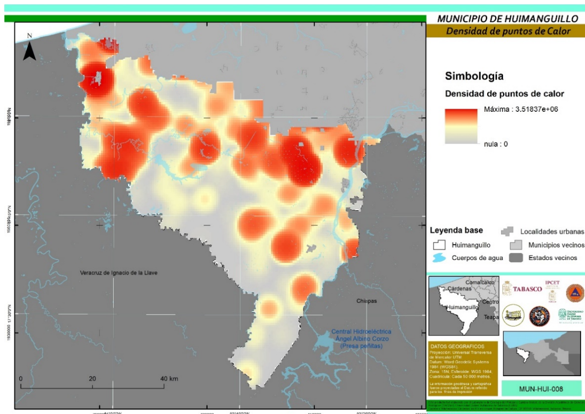
Figura 51. Focos de calor en Huimanguillo modelados a partir de los datos de las figuras 49 y 50 de enero a junio del 2024.
