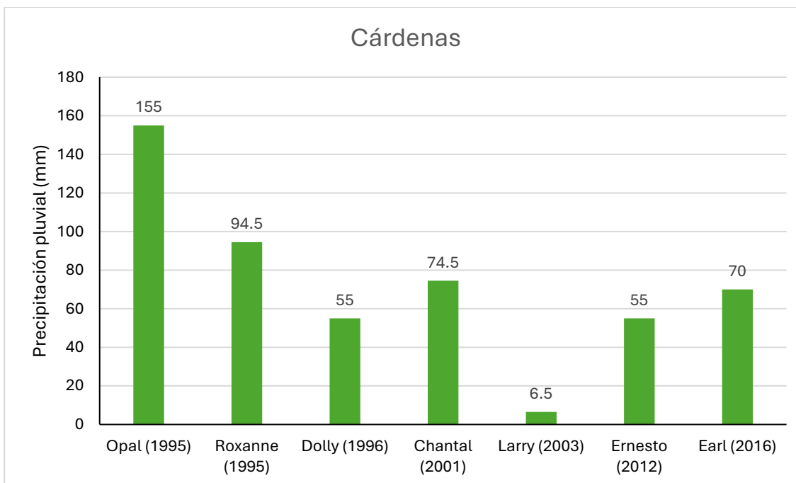
Figura 42. Precipitación pluvial máxima en 24 horas registrada para el municipio de Cárdenas originada por diversos ciclones tropicales que afectaron a Tabasco.
