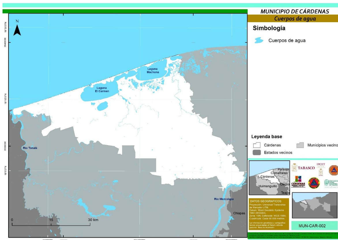
Figura 26. Cuerpos de agua que se encuentran o transitan por el municipio de Cárdenas.
