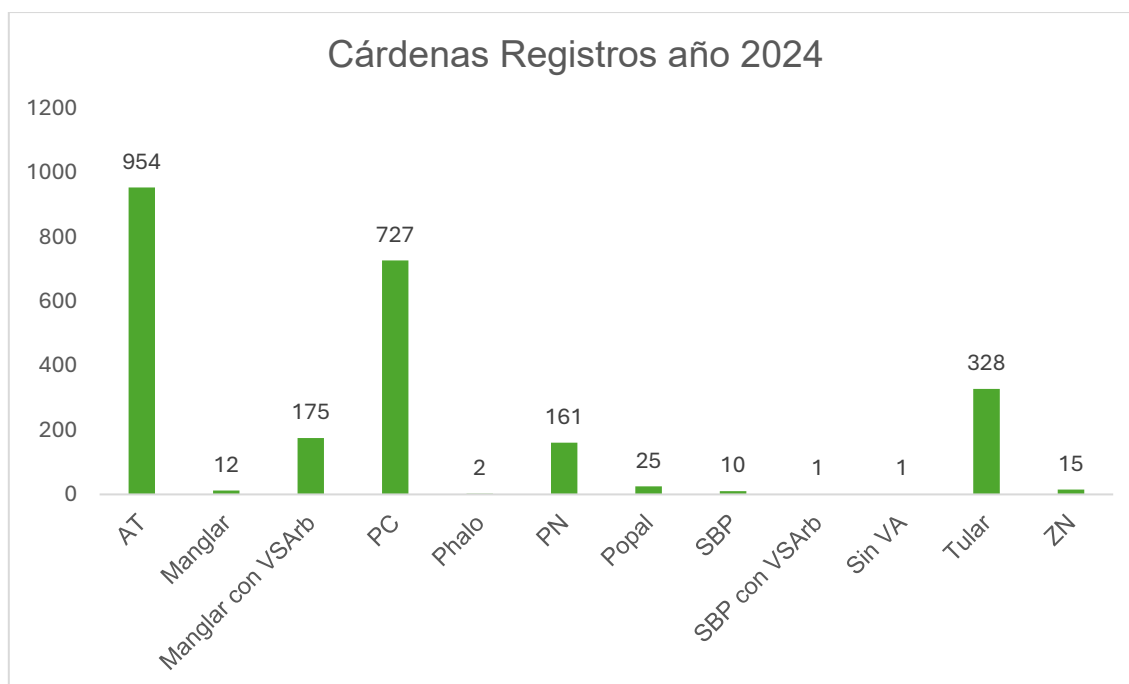
Figura 52. Gráfico con los datos de distribución de los puntos de calor de enero a junio del 2024 en los diferentes tipos de vegetación y uso del suelo 10 del municipio de Cárdenas.
