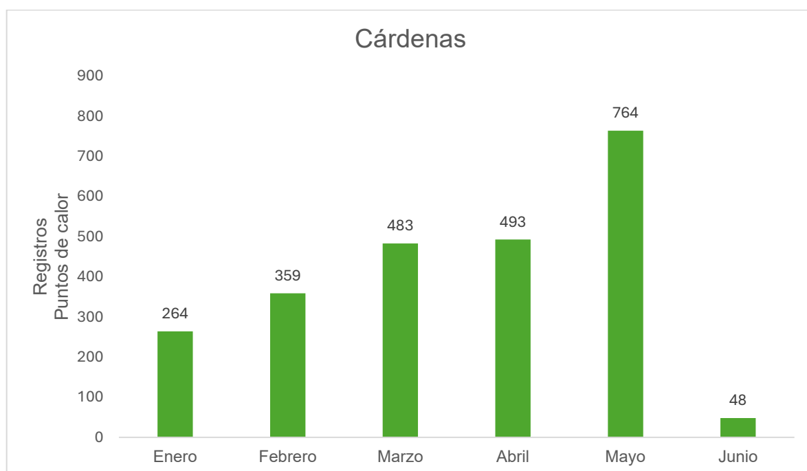
Figura 53. Gráfico con la distribución mensual de los puntos de calor para los meses de enero a junio del 2024.
