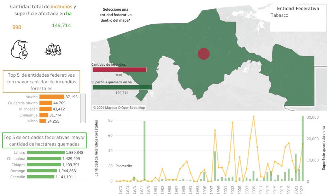
Figura 44. Datos de incendios registrados de 1970 a 2023, tomada del Sistema de Predicción de Peligro de Incendios Forestales.
