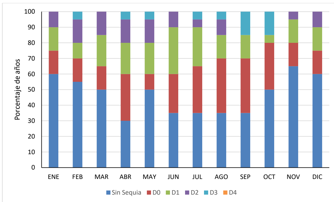
Figura 37. Ocurrencia estacional (mensual) de las condiciones de sequía en el periodo de 2003-2022. Municipio de Cárdenas, Tabasco.
