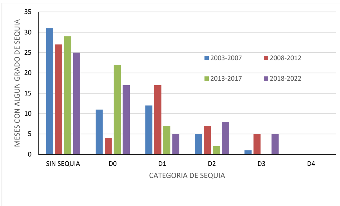
Figura 36. Ocurrencia de diversas categorías de sequía por quinquenio en el periodo de 2003-2022. Municipio de Cárdenas, Tabasco.
