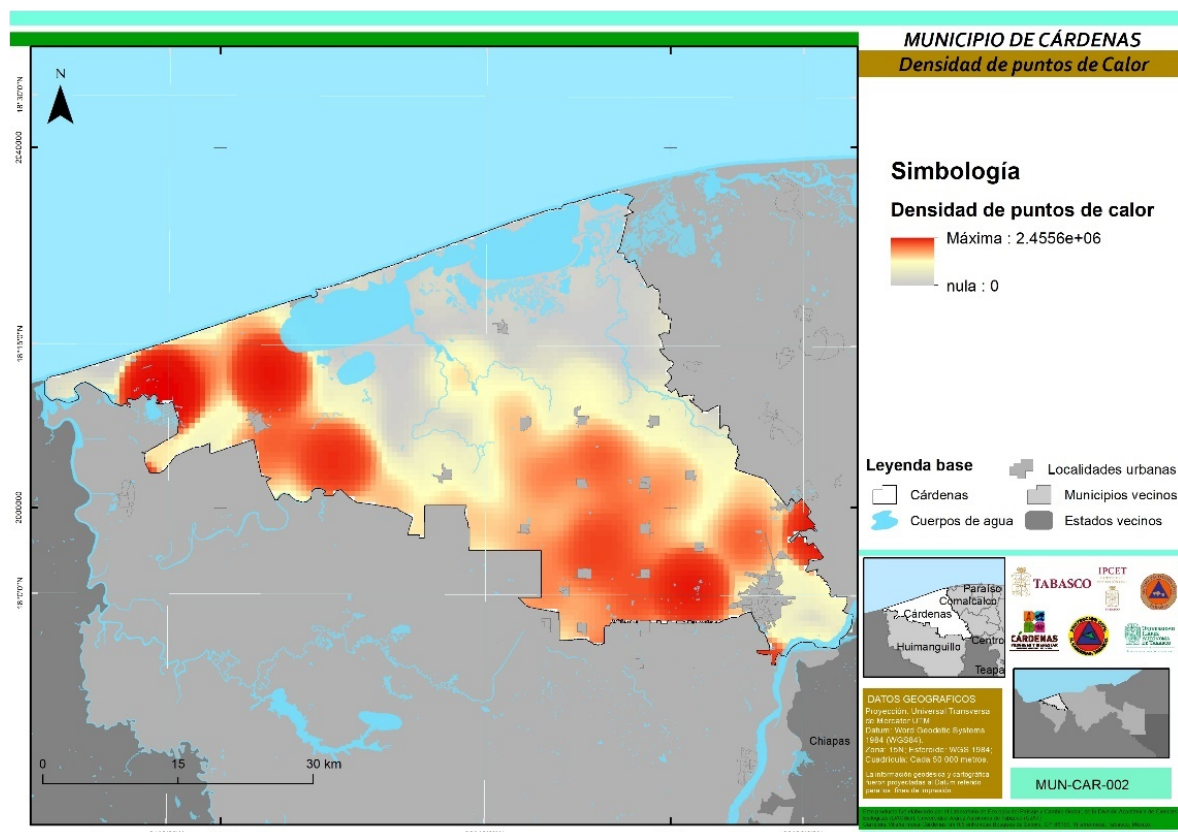
Figura 51. Focos de calor en Cárdenas modelados a partir de los datos de las figuras 49 y 50 de enero a junio del 2024.
