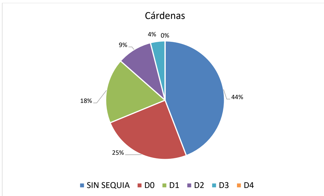
Figura 35. Frecuencia de meses con algún grado de sequía en el periodo de 2003-2022. Municipio de Cárdenas, Tabasco.
