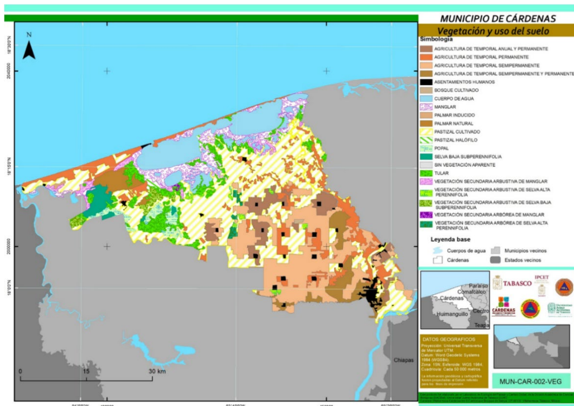
Figura 5. Mapa de Vegetación y Uso del suelo del municipio de Cárdenas.
