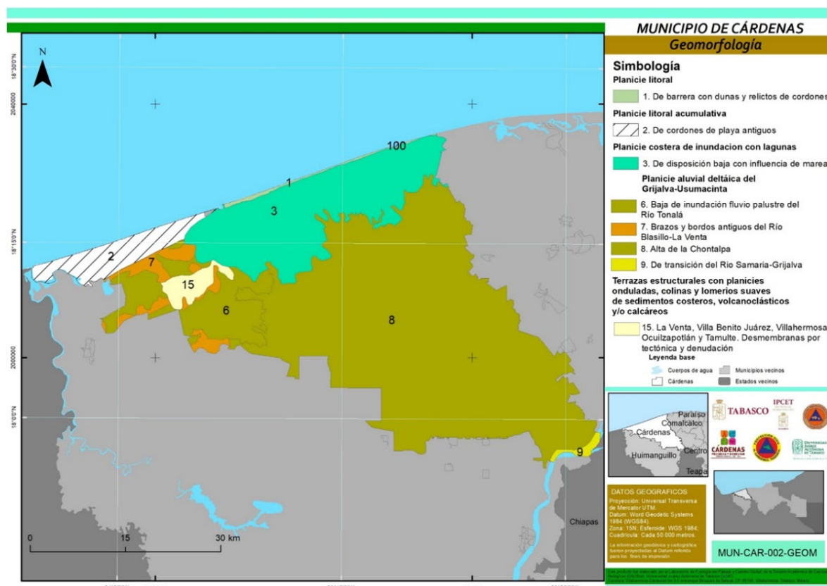
Figura 3. Mapa de Geomorfología del Municipio de Cárdenas.
