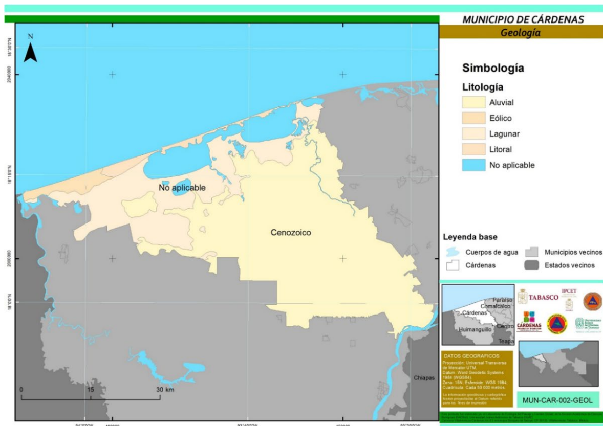
Figura 2. Mapa Geológico de Cárdenas.
