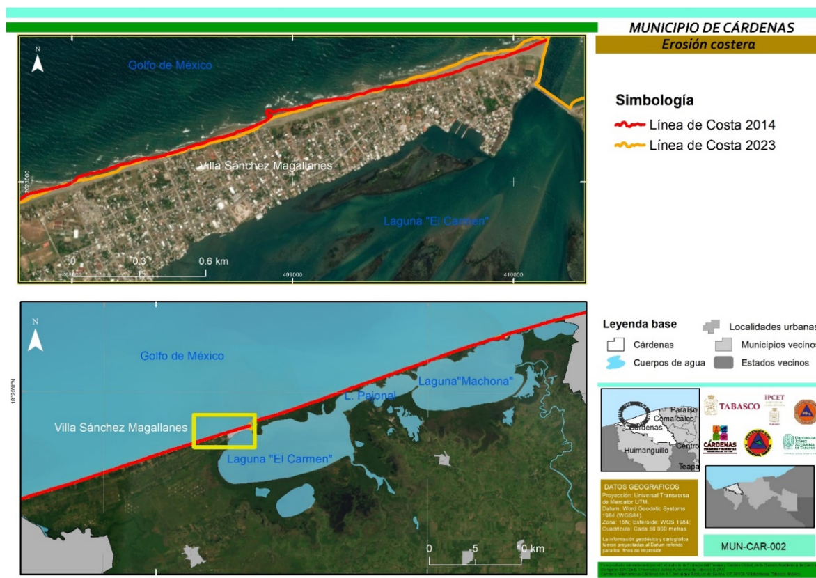
Figura 25. Zonas que evidencia el retroceso de la línea de costa en el municipio de Cárdenas.
