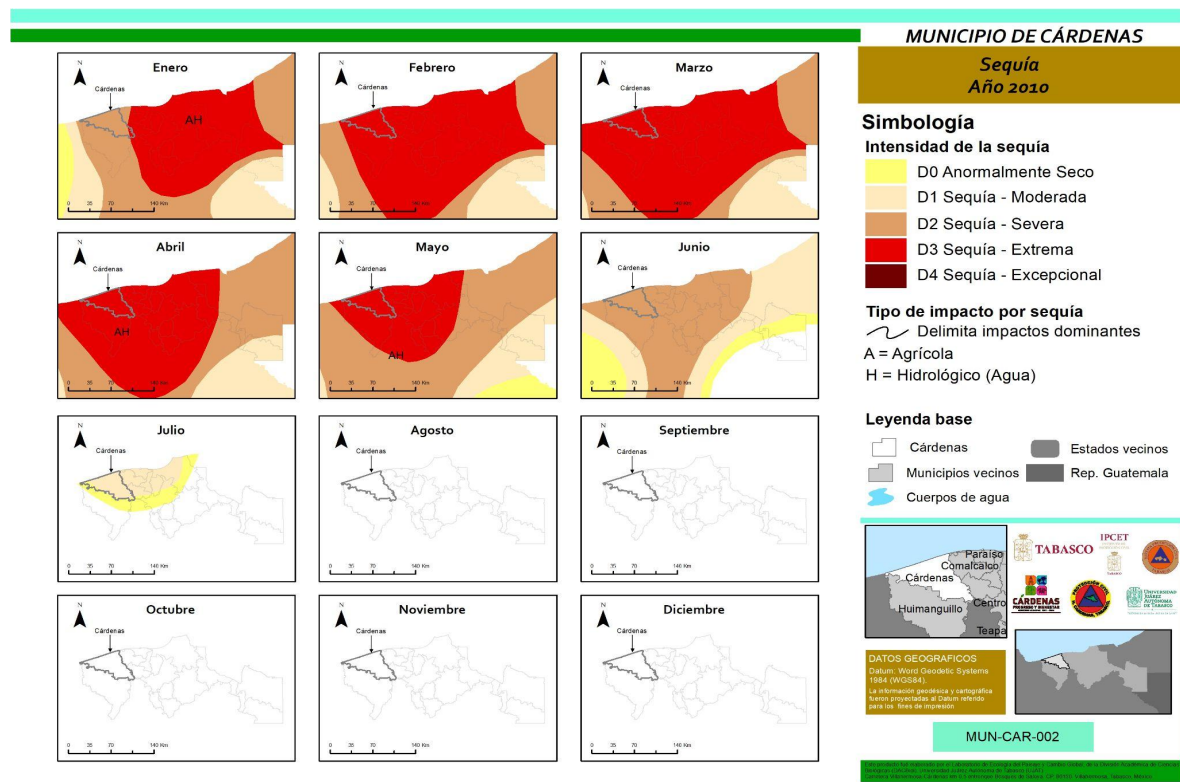
Figura 39. Categorías de sequía en el municipio de Cárdenas durante los meses del año 2010.
