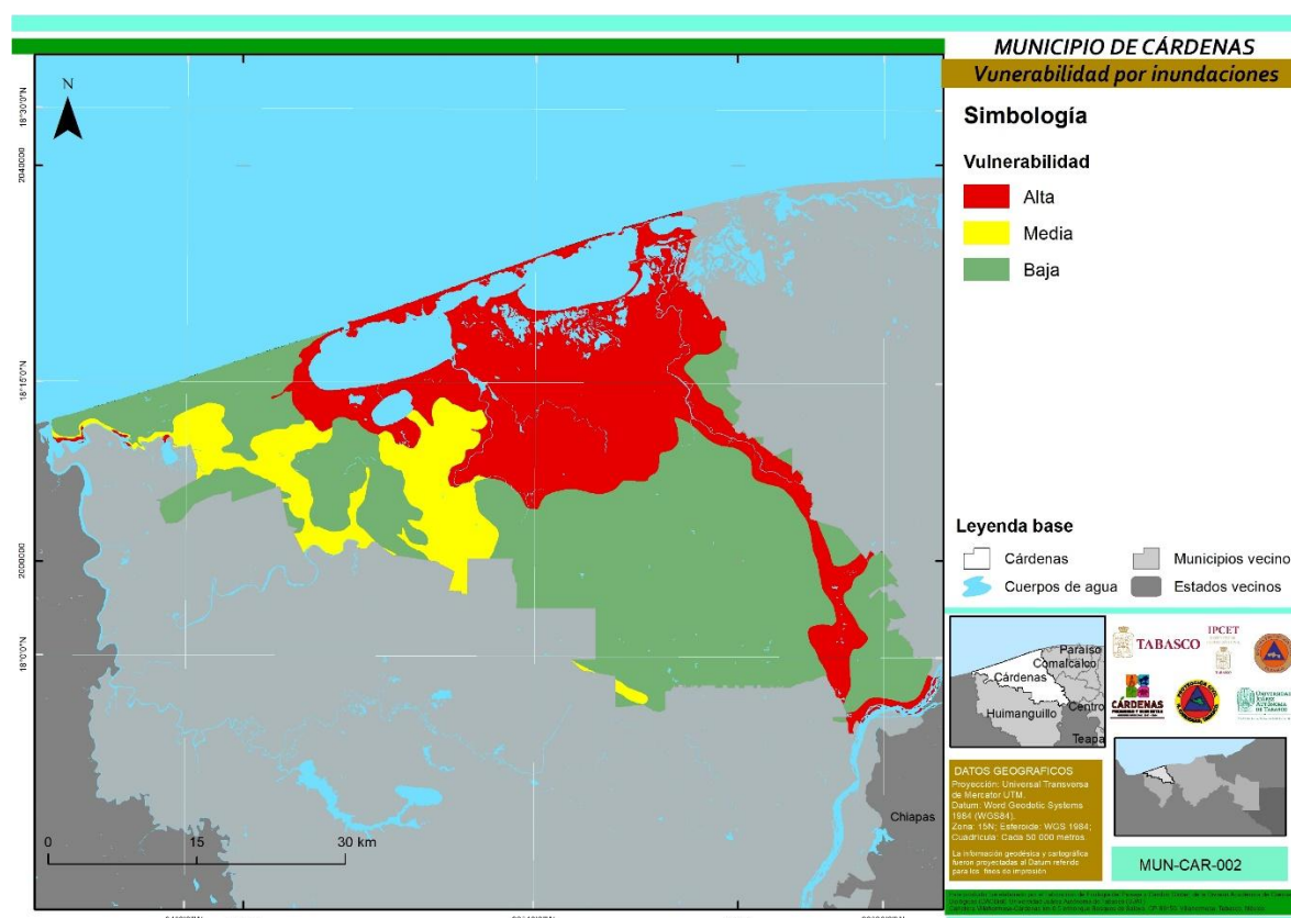
Figura 30. Zonificación del grado de vulnerabilidad a inundaciones en el municipio de Cárdenas.
