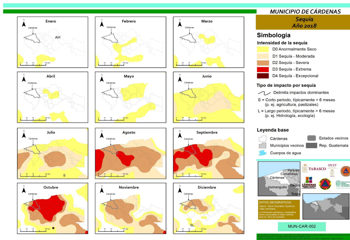
Figura 40. Categorías de sequía en el municipio de Cárdenas durante los meses del año 2018.
