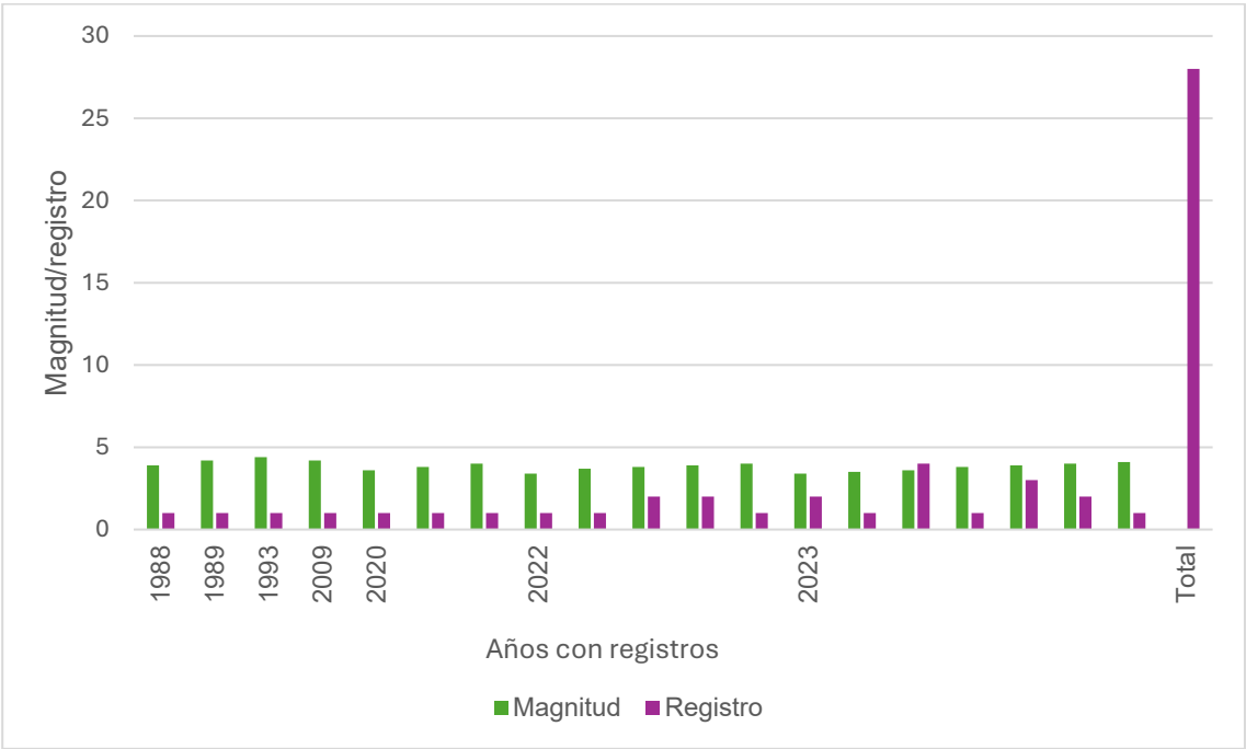
Figura 22. Gráfico con datos comparativos (magnitud/cantidad) de los sismos registrados en el municipio de Cárdenas por año.
