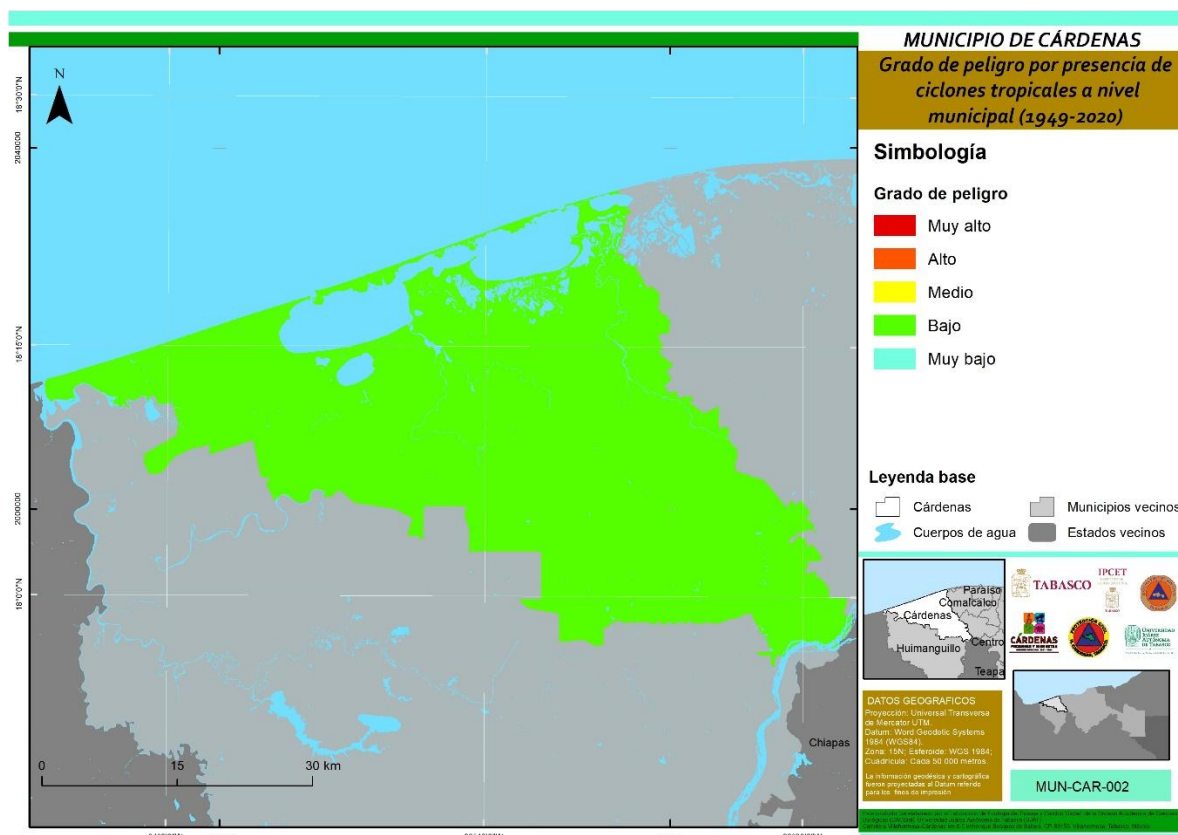
Figura 43. Grado de peligro por presencia de ciclones para el municipio de Cárdenas. Fuente: CENAPRED ( www.atlasnacionalderiesgos.gob.mx/app/mapa/?capa=vulnInund ).
