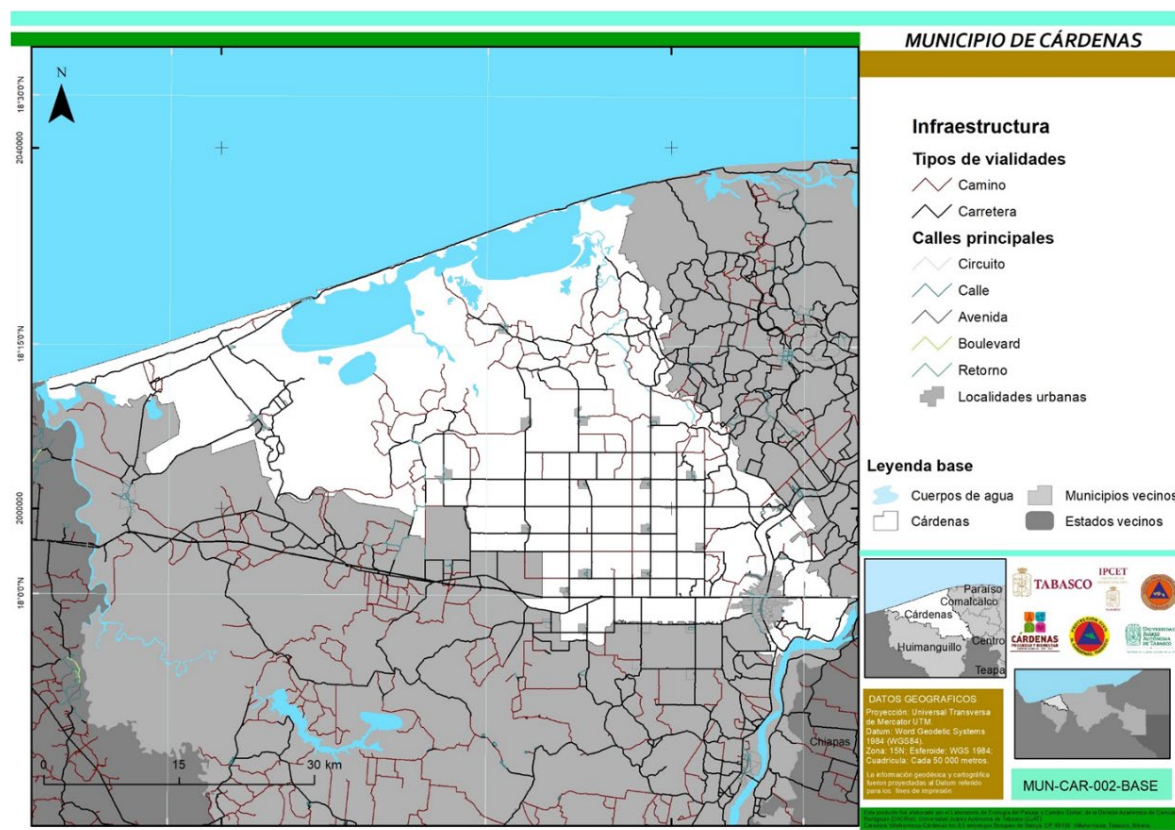
Figura 1. Mapa base del municipio de Cárdenas.
