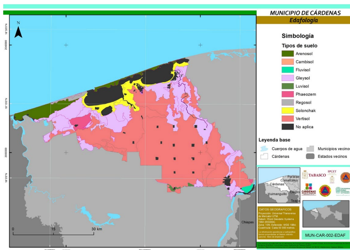
Figura 4. Mapa de la distribución de los tipos de suelos del municipio de Cárdenas.
