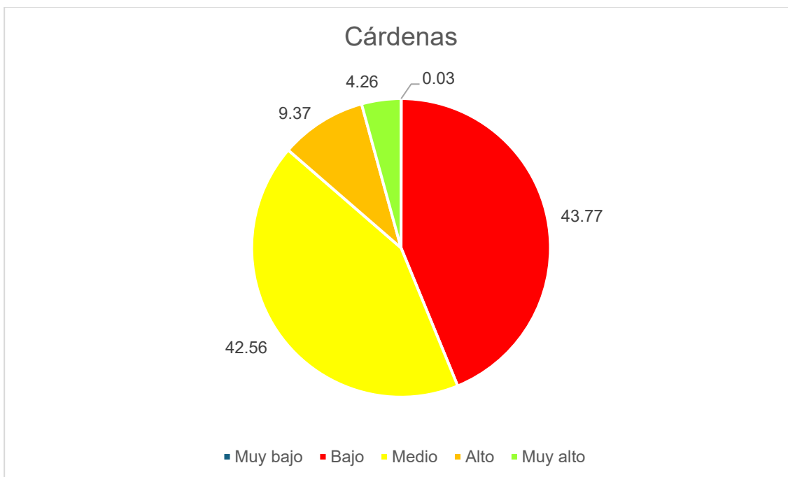
Figura 28. Proporción de la superficie municipal de Cárdenas expuesta al peligro de inundación.
