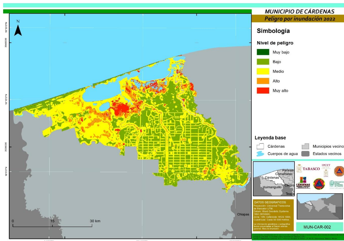
Figura 27. Zonificación del Peligro por inundaciones en el municipio de Cárdenas.
