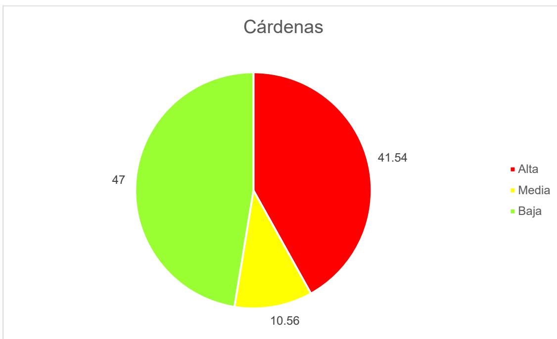
Figura 32. Proporción de la superficie municipal de Cárdenas vulnerable a la inundación.
