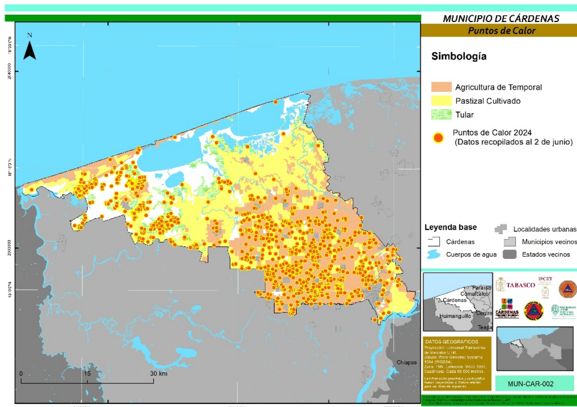
Figura 49. Mapa del municipio de Cárdenas con los datos de puntos de calor de enero a junio del 2024.
